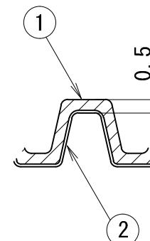
A部詳細 (尺度5/1)
